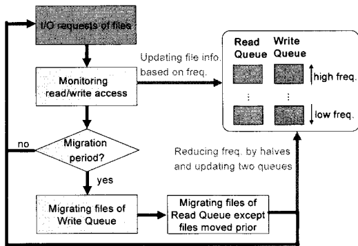
그림 1. PB-PDC의 전체 수행 흐름 Fig. 1. Overall Execution Flow of PB-PDC
