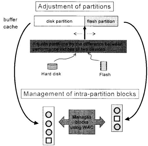
그림 2. DAC 알고리즘의 구조. DAC는 2 수준으로 구성됨: 1) 구획 조정 부분 2) 구획 내부의 블록 관리 부분
