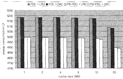
그림 5. 4개 캐시 조합의 부하 분산 알고리즘의 에너지 소모 (trace1) Fig. 5. Energy consumptions of 4 combinatory pairs of load distribution algorithms (trace1)
