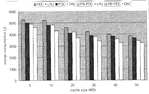
그림 7. 4개 캐시 조합의 부하 분산 알고리즘의 에너지 소모 (trace2) Fig. 7. Energy consumptions of 4 combinatory pairs of load distribution algorithms (trace2)
