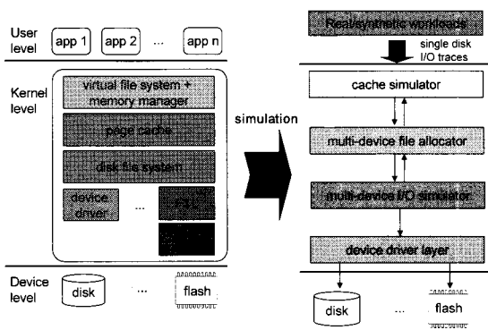
그림 3. 하드 디스크와 플래시 메모리의 쌍으로 구성된 이종 저장장치를 위한 시뮬레이션 구조 Fig. 3. Simulation architecture for a heterogeneous storage pair of a hard disk and a flash memory
