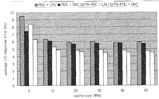
그림 6. 4개 캐시 조합의 부하 분산 알고리즘의 평균 I/O 응답 시간 (trace2) Fig. 6. Average I/O response times of 4 combinatory pairs of load distribution algorithms (trace2)
