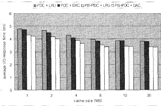
그림 4. 4개 캐시 조합의 부하 분산 알고리즘의 평균 I/O 응답 시간 (trace1) Fig. 4. Average I/O response times of 4 combinatory pairs of load distribution algorithms (trace1)
